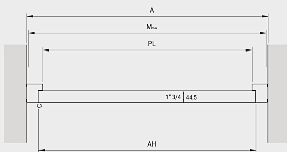
Sección horizontal
